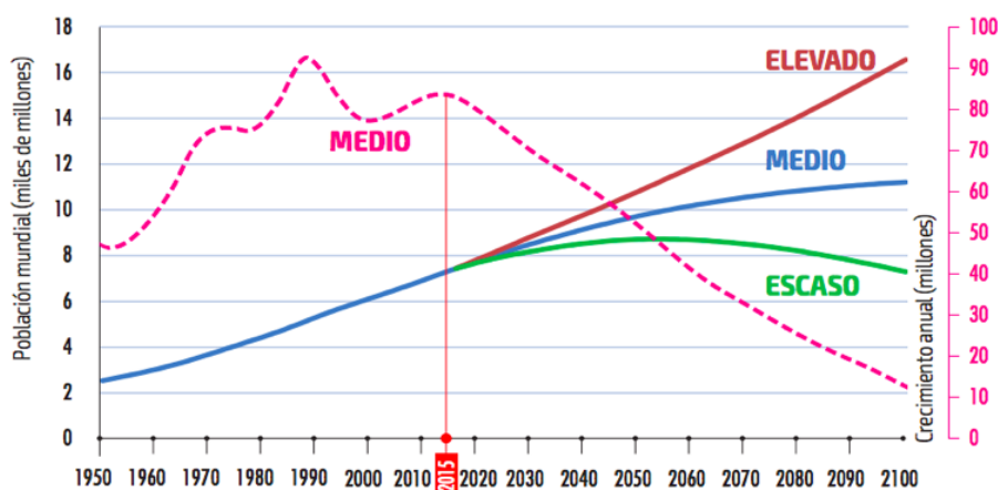
FIGURA 4. Crecimiento Demográfico Mundial hasta 2100, por variante Fuente: World Population Prospects: 2015 revisions (FAO, 2017, p.9)
