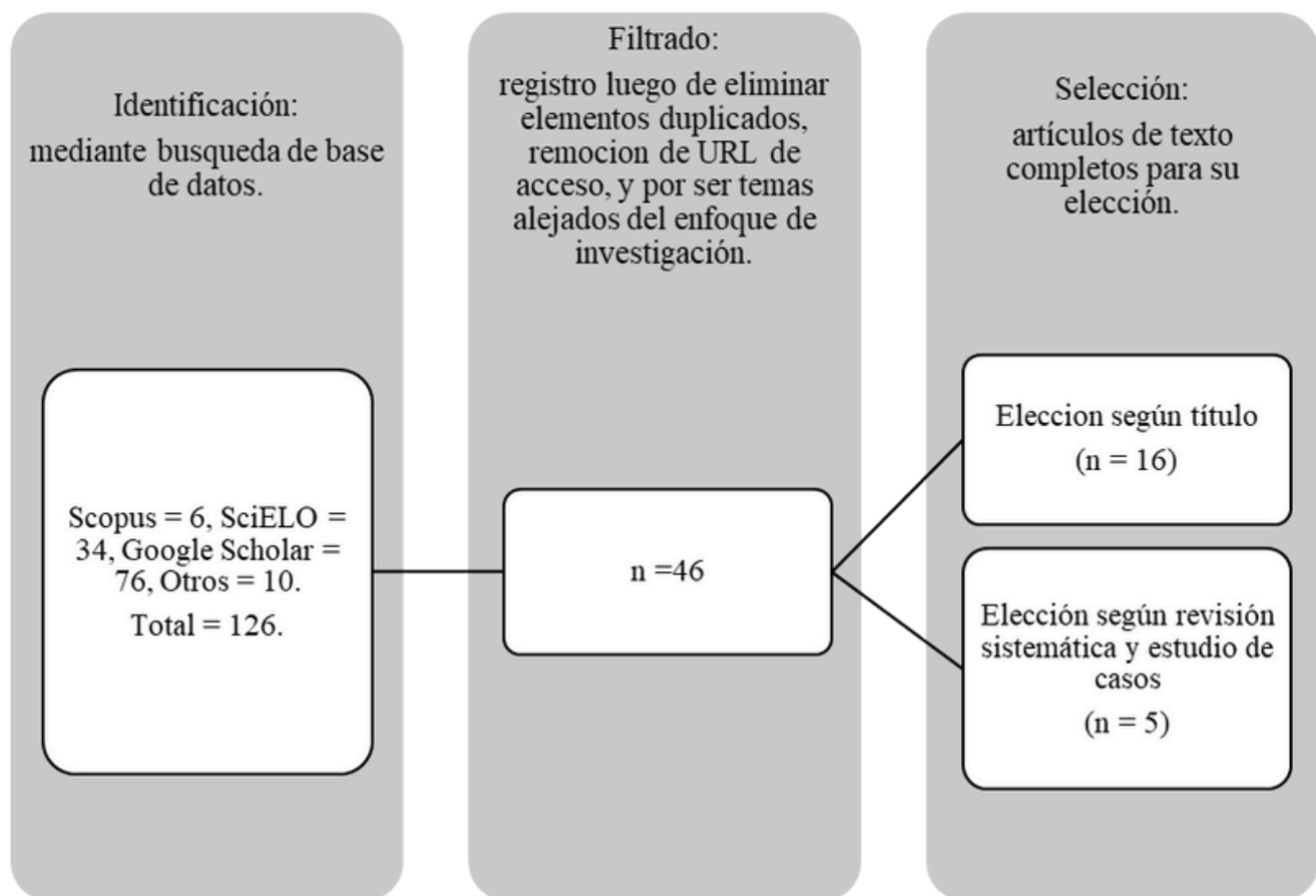
Figura 1 – Esquema PRISMA
