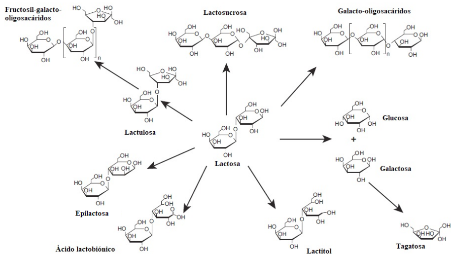
Figura 3. Estructura química de oligosacáridos no digeribles derivados de lactosa.
