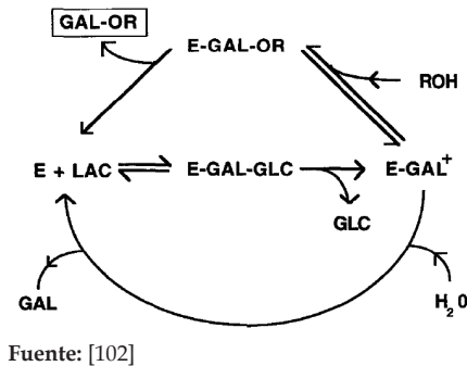
Figura 5. Mecanismo de reacción propuesto para la acción de la \beta -galactosidasa en lactosa: E: enzima; LAC: lactosa; GAL: galactosa; GAL + : estado de transición del ión carbonio; GLC: glucosa; ROH: azúcar aceptor; GAL-OR: azúcar galactosil (oligosacáridos).
