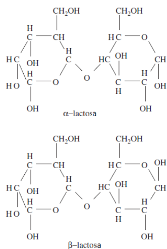
Figura 1. Estructura de la lactosa en las configuraciones \alpha y \beta .
