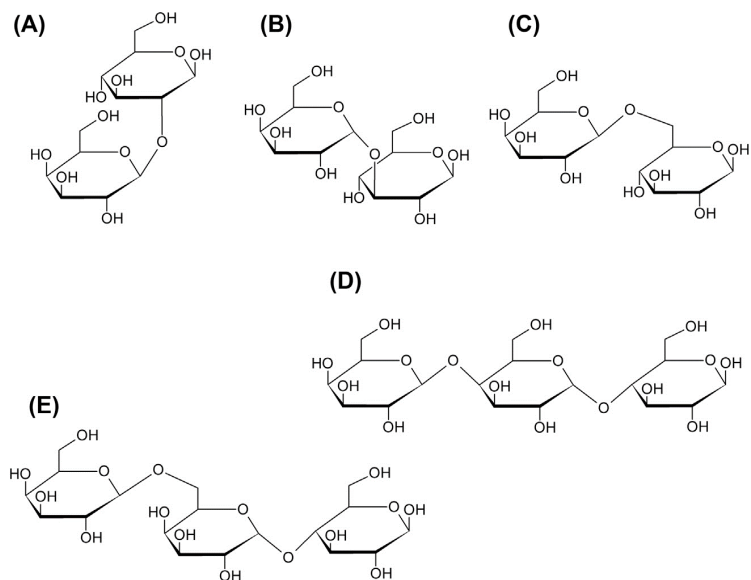
Figura 4. Estructura química de algunos galactooligosacáridos. (a) Gal(β1-2) Glu; (b) Gal(β1-3)Glu; (c): Gal(β1-6)Glu; (d): Gal(β1-4)Gal(β1-4)Glu; (e): Gal(β1-6)Gal(β1-4)Glu.
