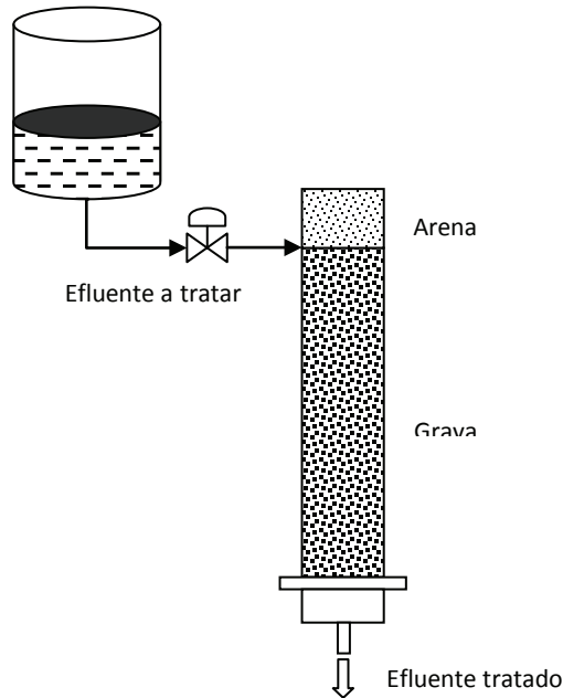
FIGURA 1. ESQUEMA DEL REACTOR
