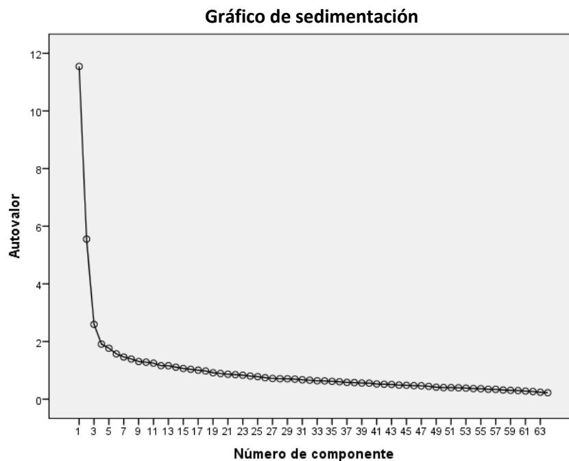
Figura 1. Gráfico de sedimentación – Extracción de factores - ERE
