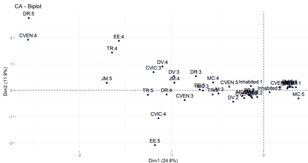
Figura 2. Proyección sobre correlaciones de localidades y MDM.
