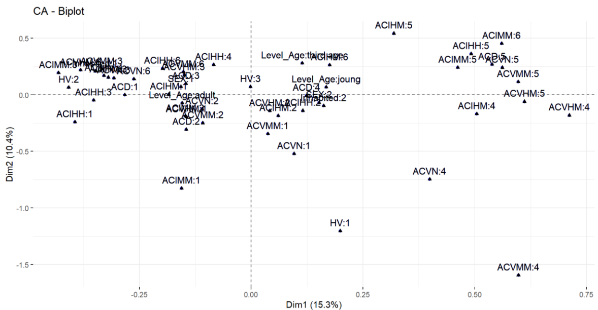
Figura 1. Proyección sobre correlaciones de localidades, Sexo, HV, Edad y AC
