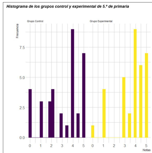
Figura 1. Histograma de los grupos control y experimental de 5.º de primaria
