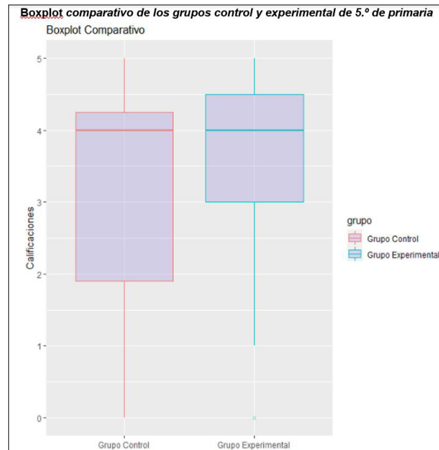
Figura 2. Boxplot comparativo de los grupos control y experimental de 5.º de primaria
