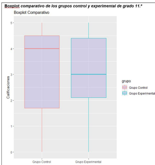
Figura 4. Boxplot comparativo de los grupos control y experimental de grado 11.º
