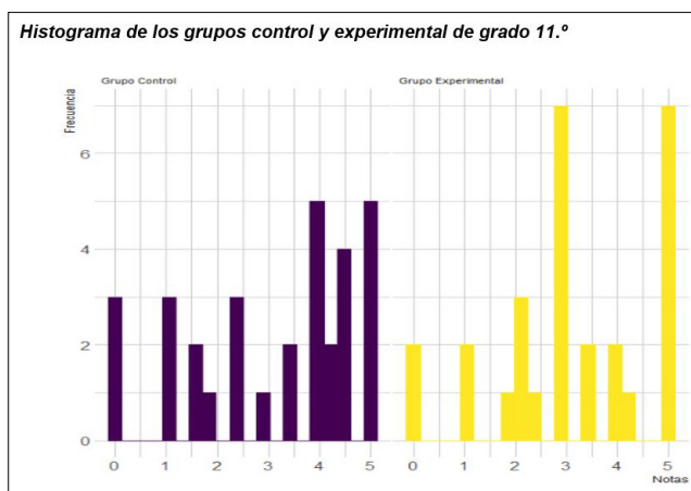
Figura 3. Histograma de los grupos control y experimental de grado 11.º
