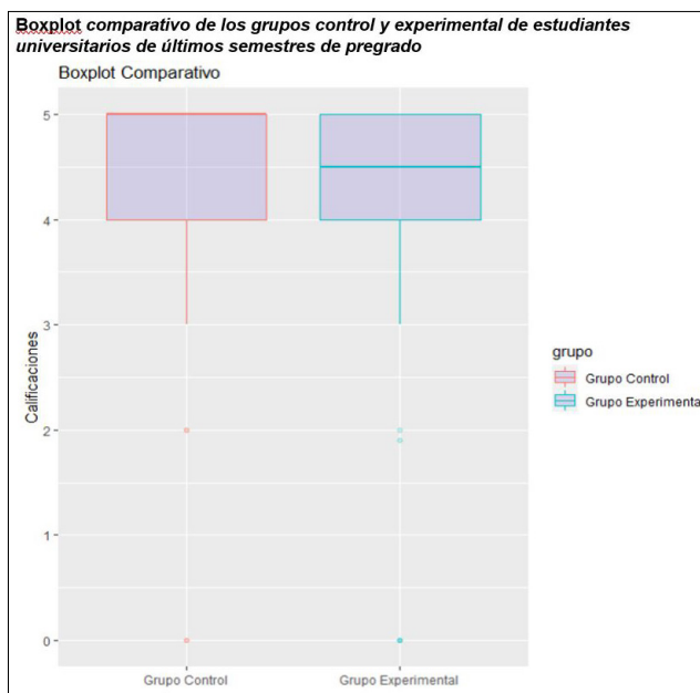
Figura 6. Boxplot comparativo de los grupos control y experimental de estudiantes universitarios de últimos semestres de pregrado
